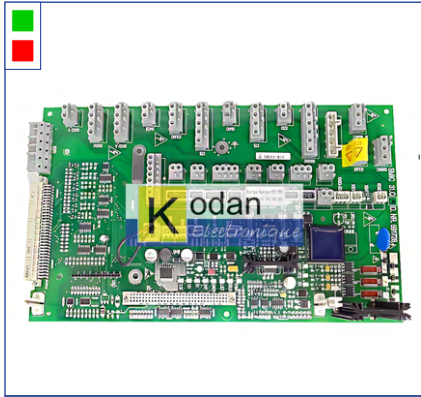
Carte porteur SMIC 31.Q (SCHINDLER)
