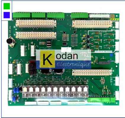
Carte porteur MCI C (THYSSEN)
