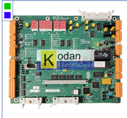
Carte de manœuvre LCE CPU40 (KONE)
