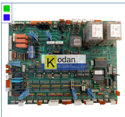
Carte de manœuvre N10(x) de A191 (AUTINOR)
