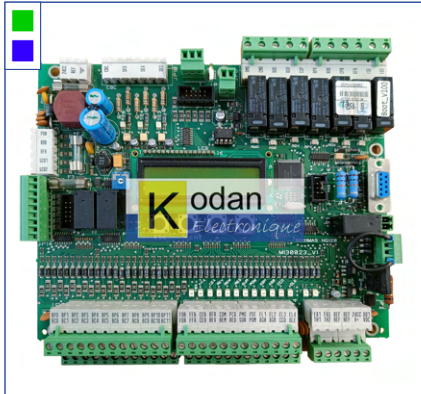
Carte de manœuvre NG120 (SODIMAS)
