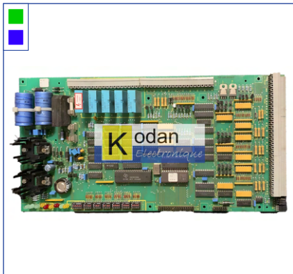
Carte de manœuvre PEG25.Q MICONIC C (SCHINDLER)
