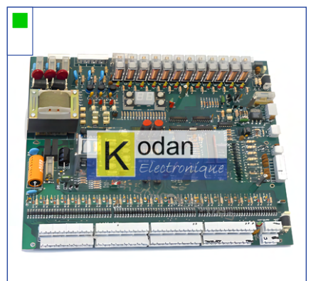
Carte de manœuvre NG02 (MEA)
