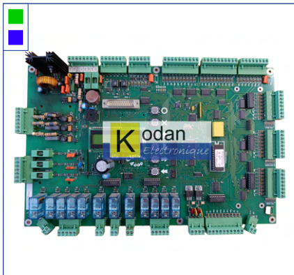
Carte de manœuvre OPTIMA 4000 (CG2A)
