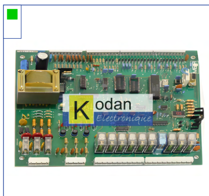
Carte de manœuvre NG01 (MEA)
