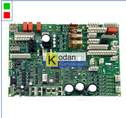
Carte de manœuvre TCBC (OTIS)
