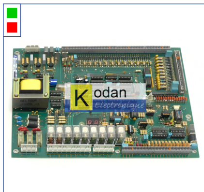
Carte de manoeuvre ICU (MEA)
