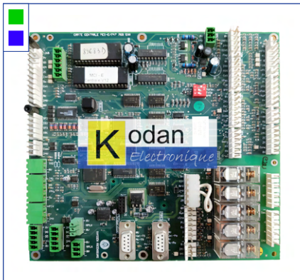
Carte de manœuvre MCI D E (THYSSEN)
