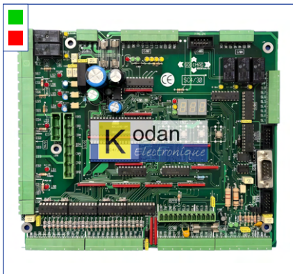
Carte de manœuvre SC4 30 (SODIMAS)
