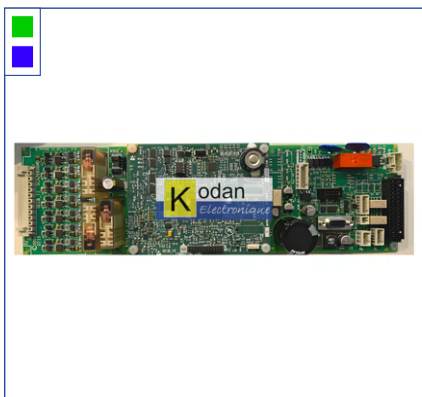
Carte de manoeuvre GECB_II (OTIS)
