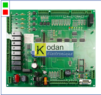
Carte de base ARCA1 (ORONA)
