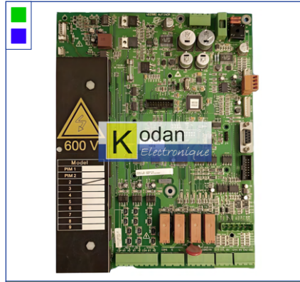
Carte de commande VF VEC50 (AUTINOR)
