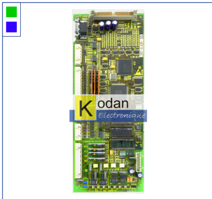
Carte de commande de VF MCB II (OTIS)
