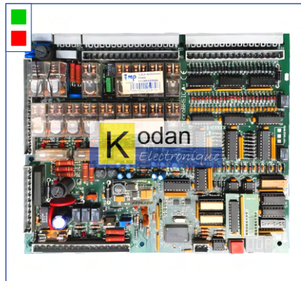
Carte de manœuvre MICROBASIC (MACPUARSA)
