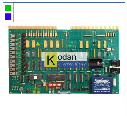
Carte de manoeuvre KFEB14.Qx (SCHINDLER)
