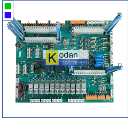
Carte porteur TYPE S (SORETEX)
