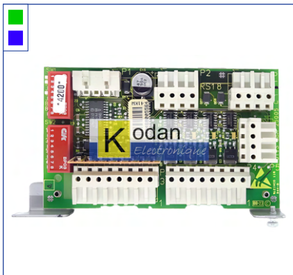
Carte remote RS18 (OTIS)
