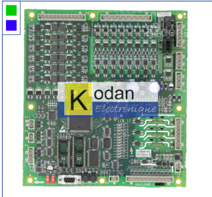
Carte de manœuvre LCBI D1 (MCS200) (OTIS)
