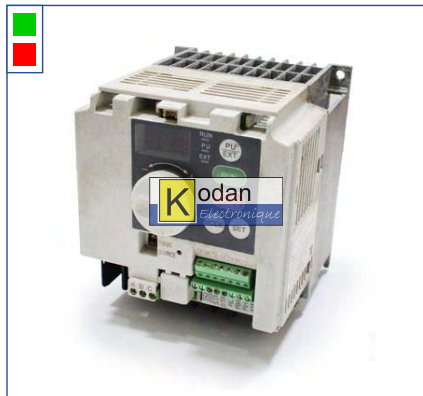
VF Mitsubishi Fr S540 075K Ec
