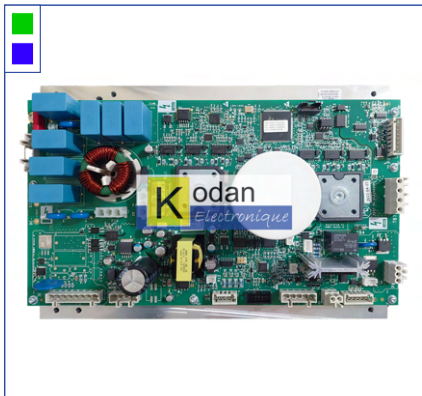
Carte pour ReGen DCPB Drive Control Power Board (OTIS)
